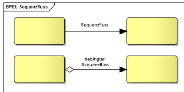
Bild 4-7: BPEL Sequenzfluss
