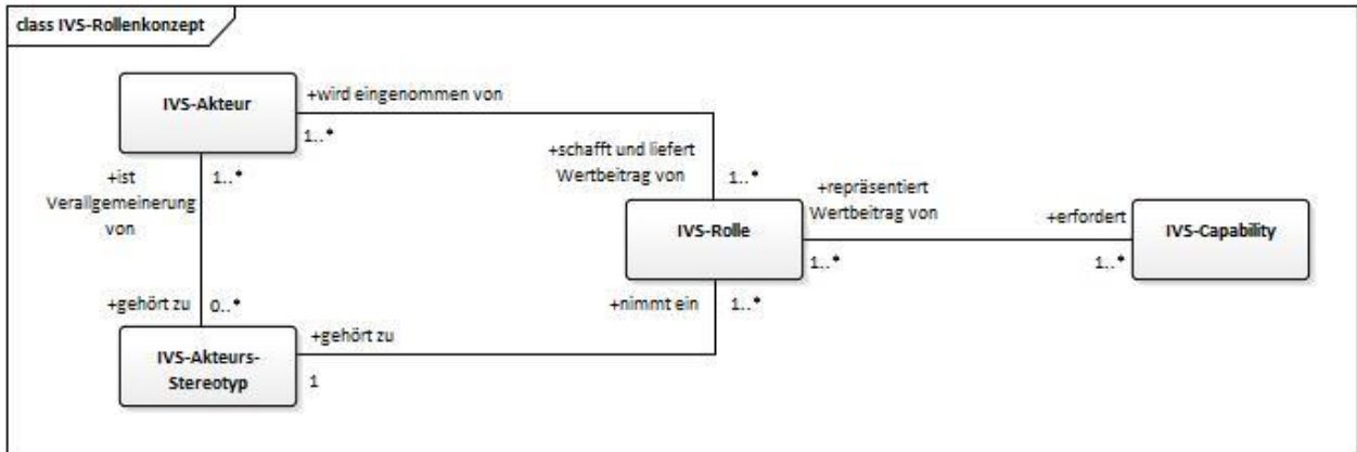
Bild 3-2: IVS-Rollenkonzept als UML-Diagramm
